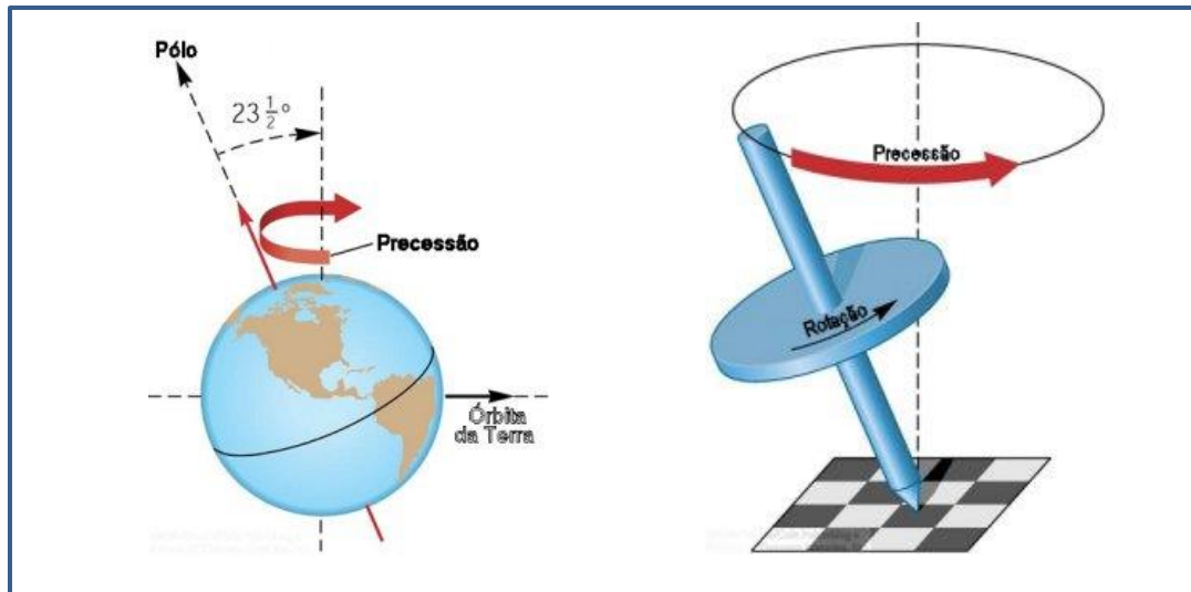
Figura 10 – Movimento de precessão da Terra (Fonte: Fonte: SILVA, José G.R. Ciclos Orbitais ou Ciclos de Milankovitch. Textos de Glossário Geológico Ilustrado. 2007. p. 1.)
