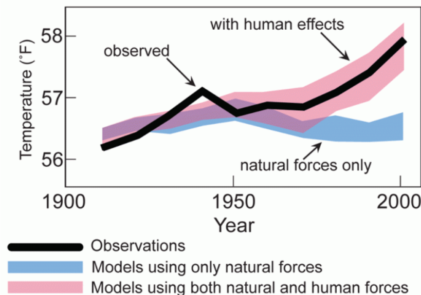
Figura 3 – Comparação das mudanças observadas na temperatura da superfície em escalas continental e global (Fonte: IPCC - Intergovernmental Panel on Climate Change 2007)
