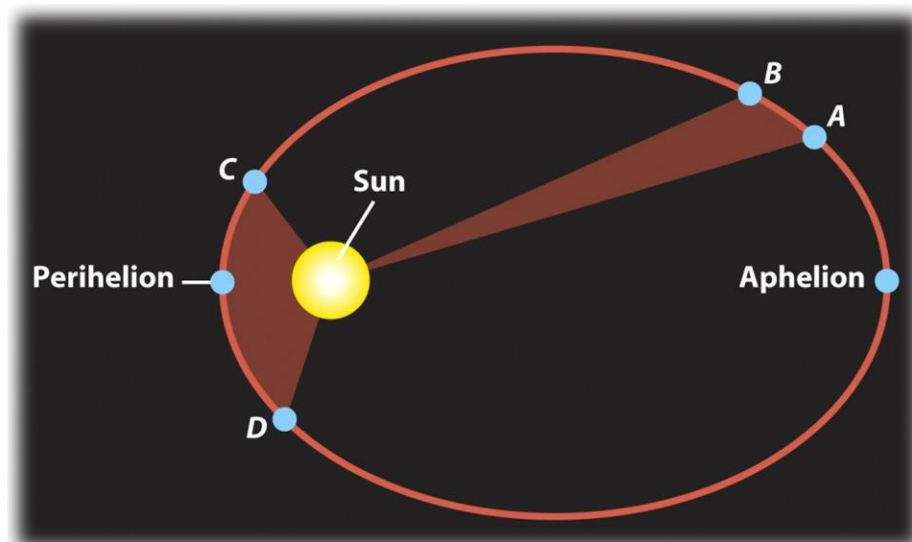
Figura 5 – Periélio e Afélio da Terra em seu movimento de translação (IPCC - Intergovernmental Panel on Climate Change 1990)
