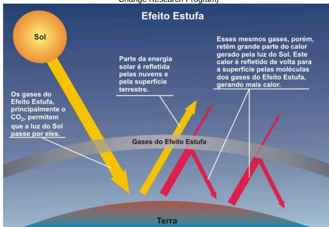
Figura 2 – Esquema do efeito estufa na Terra (Fonte: adaptado de Efeito Estufa, U.S. Global Change Research Program)
