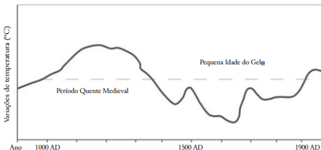
Figura 1 – Curva de variações de temperaturas durante o último milênio (Fonte: IPCC - Intergovernmental Panel on Climate Change 1990)
