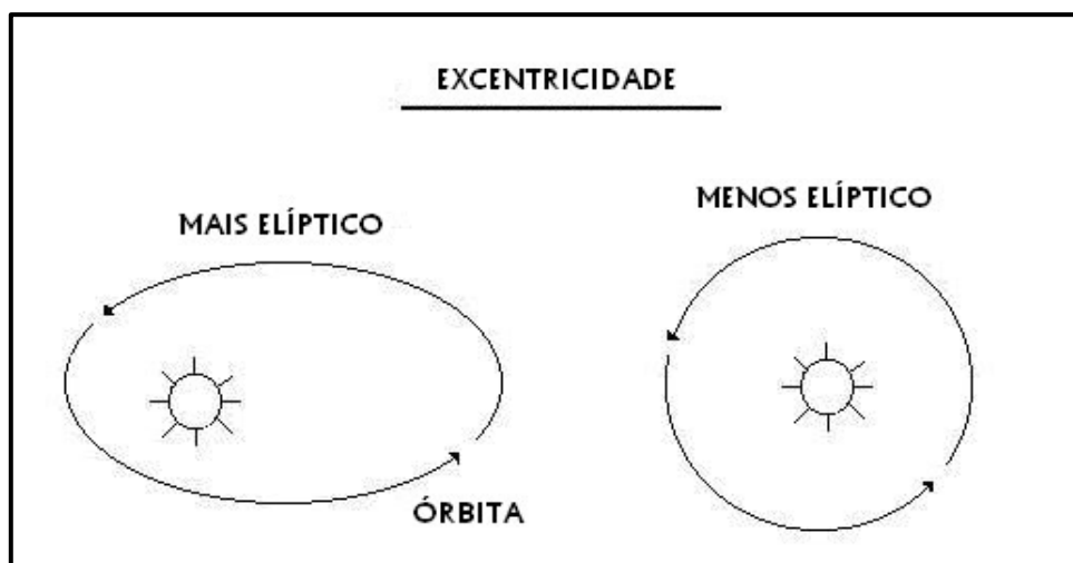
Figura 9 – Órbita elíptica mais excêntrica e órbita elíptica menos excêntrica (Fonte: CANALLE, J. - Revista Geouerj, p. 76, 1998)
