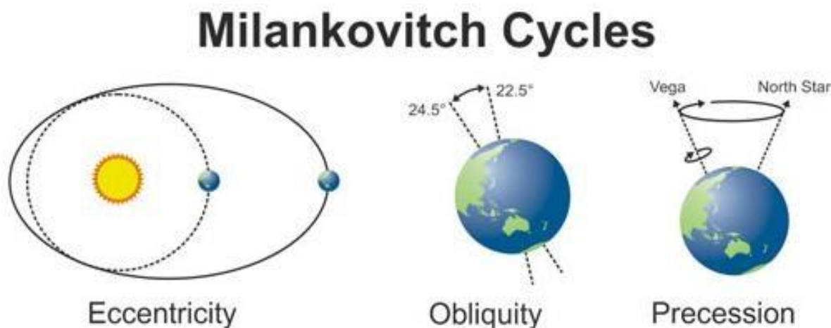
Figura 8 – Ciclos de Milankovitch movimentos que interferem no macro clima Planetário (Fonte: https://sites.google.com/site/greenprojectcom/Pgina-inicial/alteracoes-climaticas-antropogenicas ).
