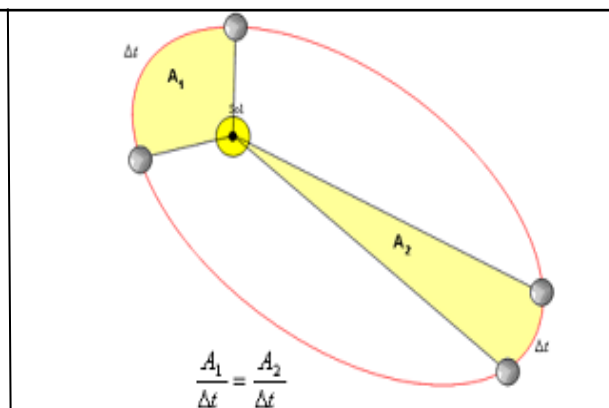
Figura 7 – Lei das áreas (IPCC Intergovernmental Panel on Climate Change 1990)
